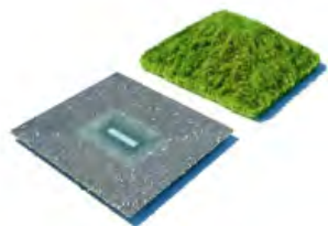
PARCO GIOCHI idelflusso acqua piovana canalizzazione idasso erba su rete di supporto
